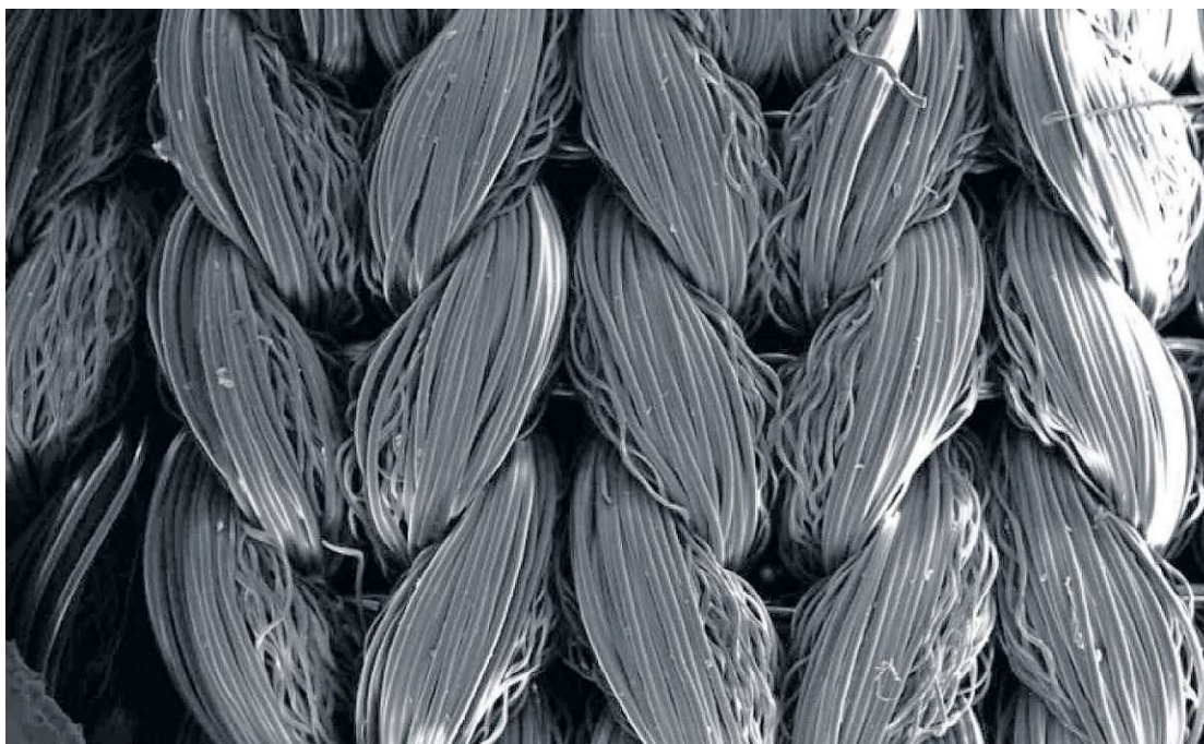
Camadas são compostas por estratos de malha de fios condutores e mudam de resistência se pressionadas
